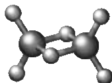
Diborane, B_2H_6
